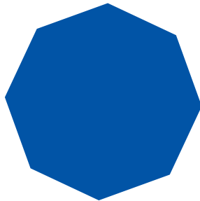
Ocatagon
