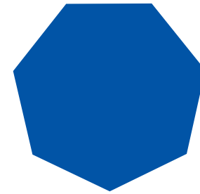
Septagon
